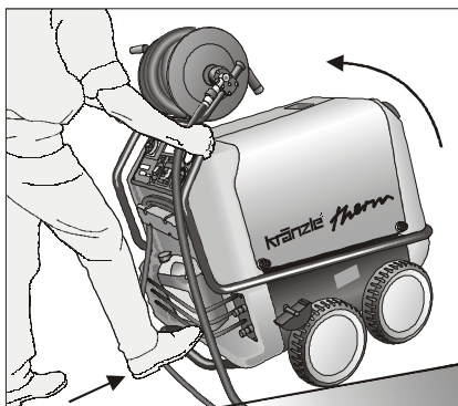
Bremse geöffnet
