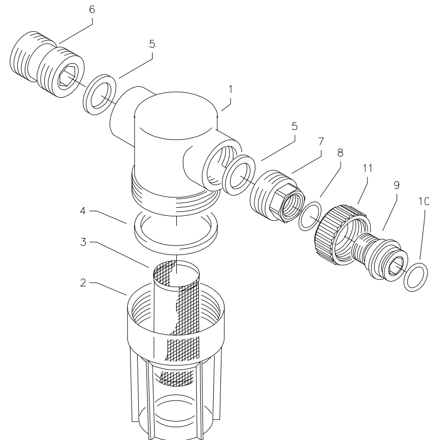
Ersatzteilliste WassereingangsfILTER
